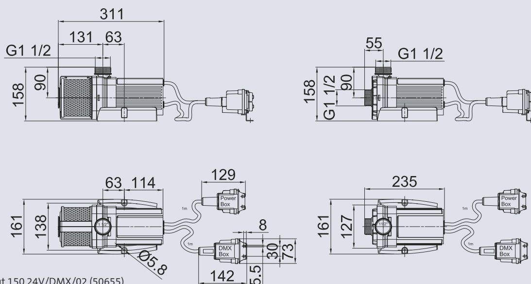
Varionaut 150 24V/DMX/02 (50655)
